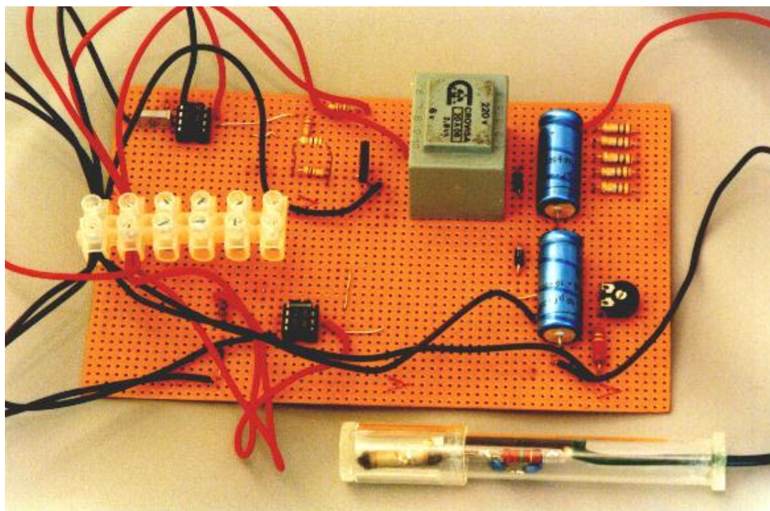
El convertidor d'alta tensió i el tub Geiger-Müller
